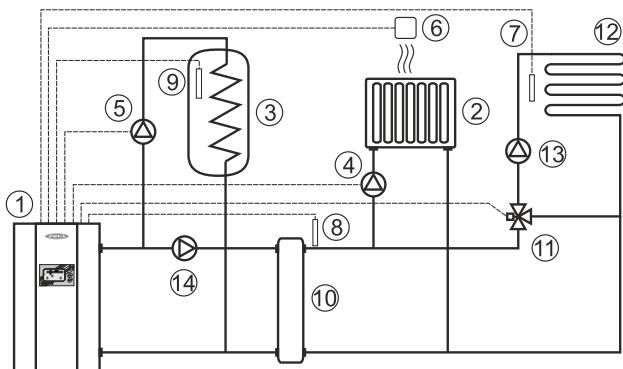
Рис.7 Упрощенная схема подключения котла с гидроразделителем, контурами ГВС и теплого пола.
