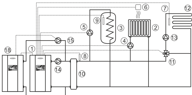
Рис.8 Упрощенная схема подключения двух котлов в каскаде с гидроразделителем, контурами ГВС и теплого пола.
