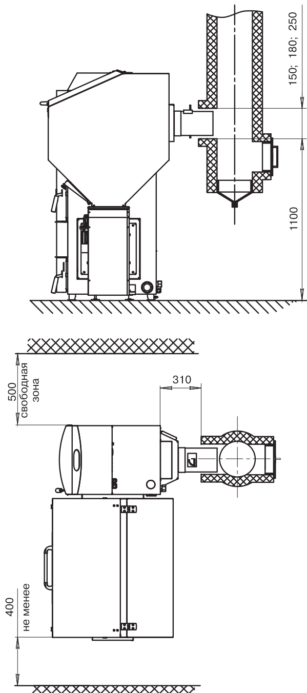
Рис.7 Схема установки котла Соединение котла с дымоходом и устройством чистки стр.10
